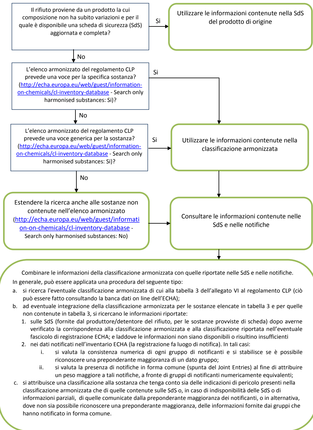
Figura 2.4 - Possibile procedura di consultazione delle fonti dei dati ai fini della classificazione dei rifiuti
